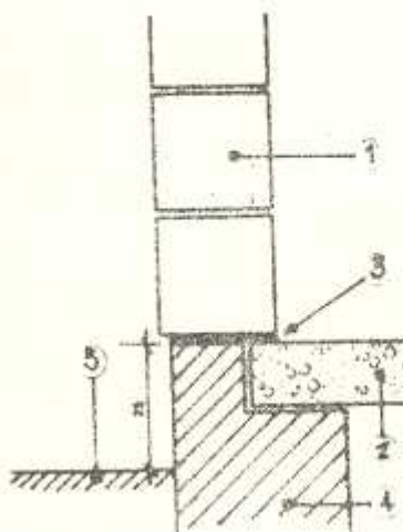
Mur plein en blocs maçonnés
