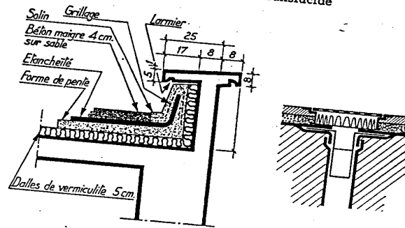
Fig. 78 — Lanterneau translucide
