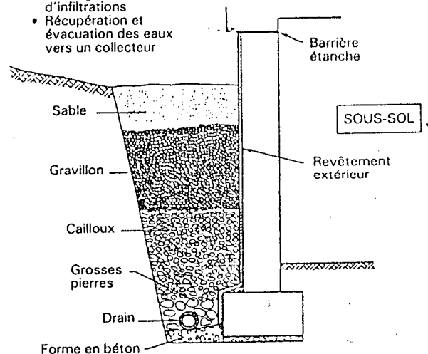
PROTECTION DES MURS ENTERRÉS (D.T.U. 20,1)
