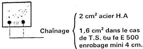
Chaînage minimal (D.T.U. 13,12)
