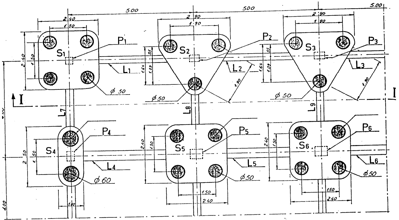
VUE EN PLAN D'UN ANGLE DE BÂTIMENT FIG. 1
