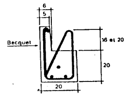
POUTRE DE RIVE (avec béquet) (doc Rector)
