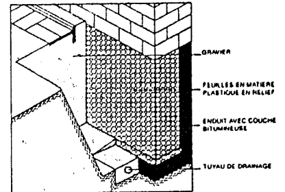
Drainage périphérique
