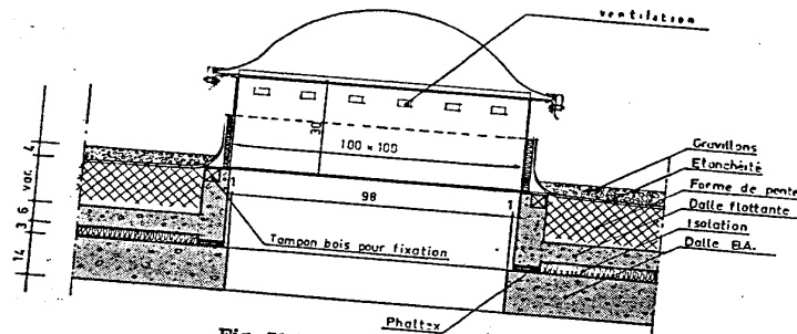
Fig. 78 — Lanterneau translucide
