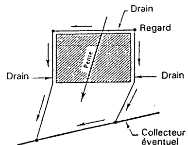
Cas des terrains en pente
