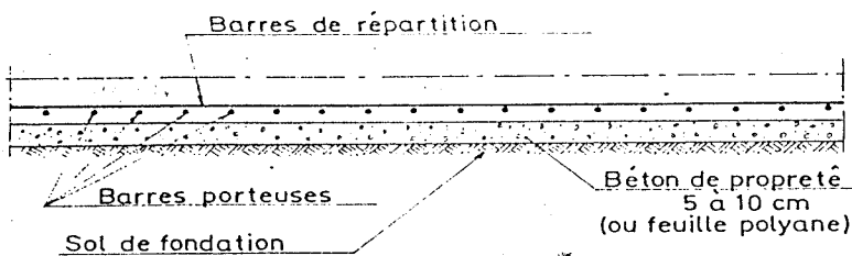
Coupe partielle longitudinale sur aciers. FIG. 27
