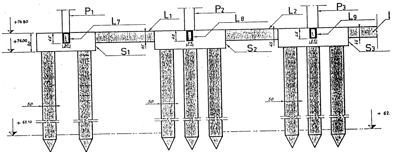
COUPE I-I FIG. 2 FONDACTIONS PAR PIEUX
