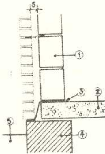
Mur composite avec lame d'air
