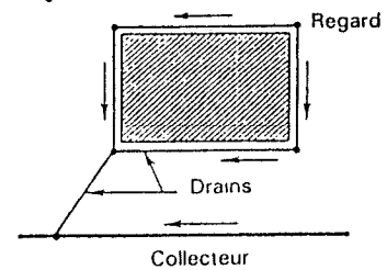
Cas des terrains sensiblement plats
